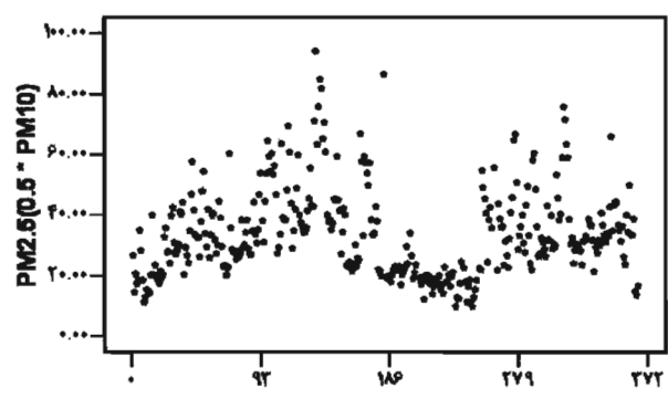
نمودار شماره ۲: پراکندگی ذرات کوچکتر از ۱۰ میکرون بر حسب غلظت ( \mu g/m^3 ) در برابر روزهای سال ۱۳۸۵
